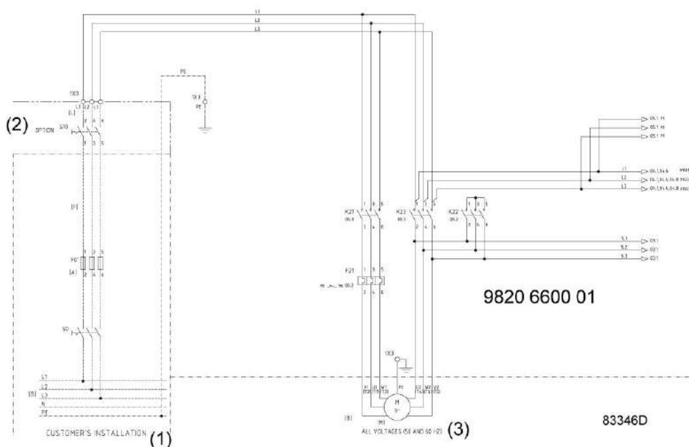
Электрические подключения для компрессоров с GA 30+ по GA 45+
