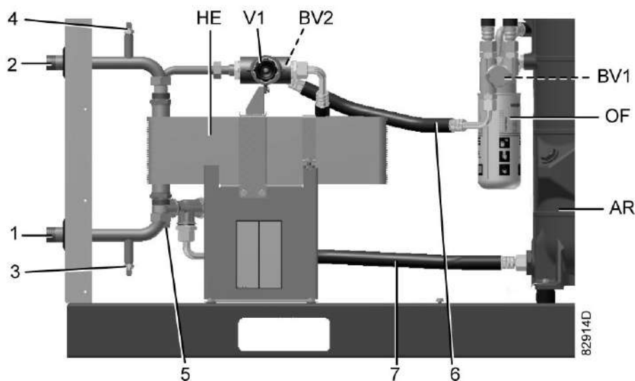
Основные компоненты блока ER
