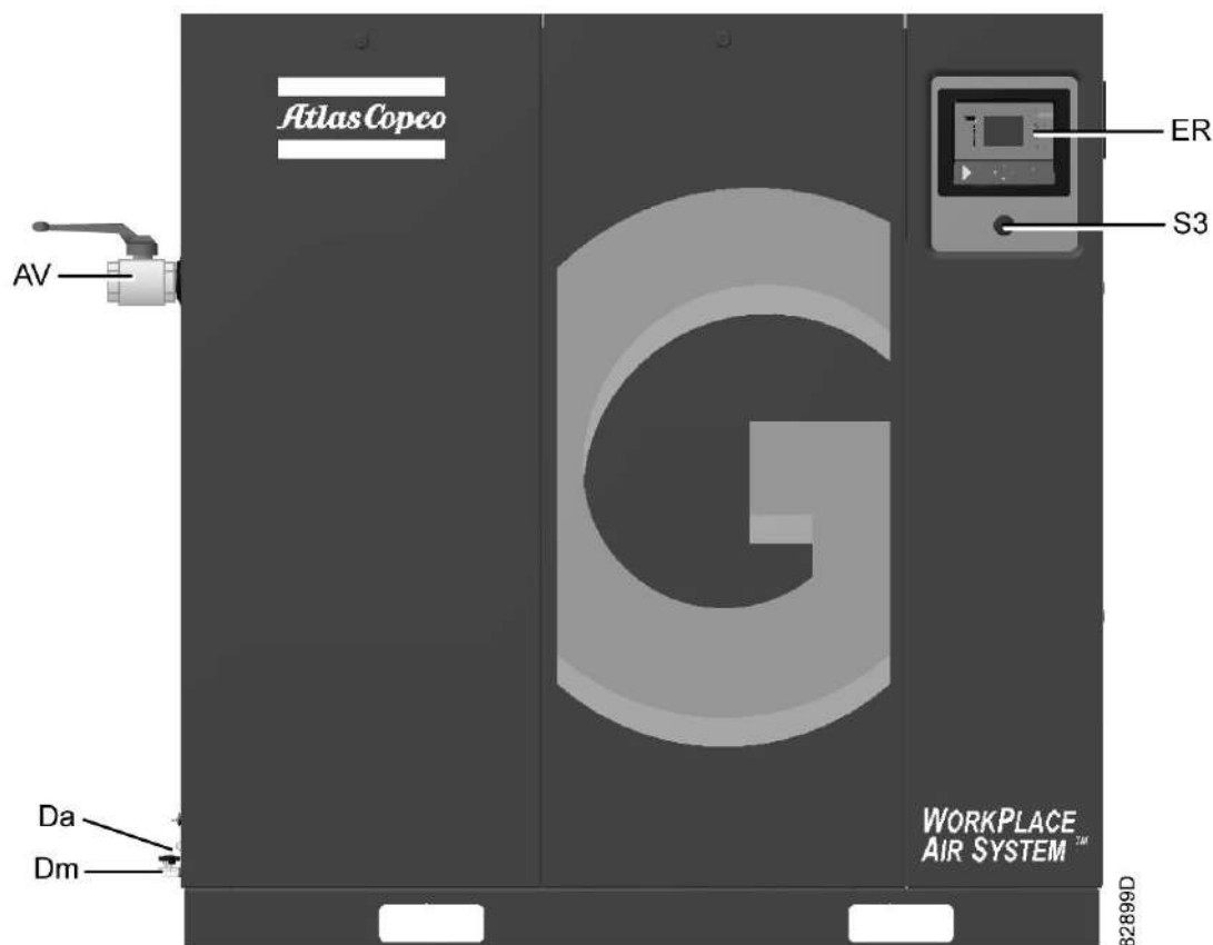
Вид спереди, компрессоры с GA 30 + по GA 45 +
