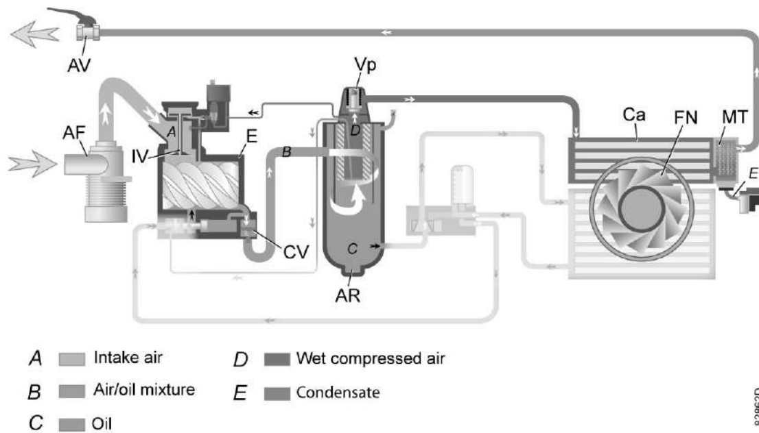
Схема потока, компрессоры GA Workplace
