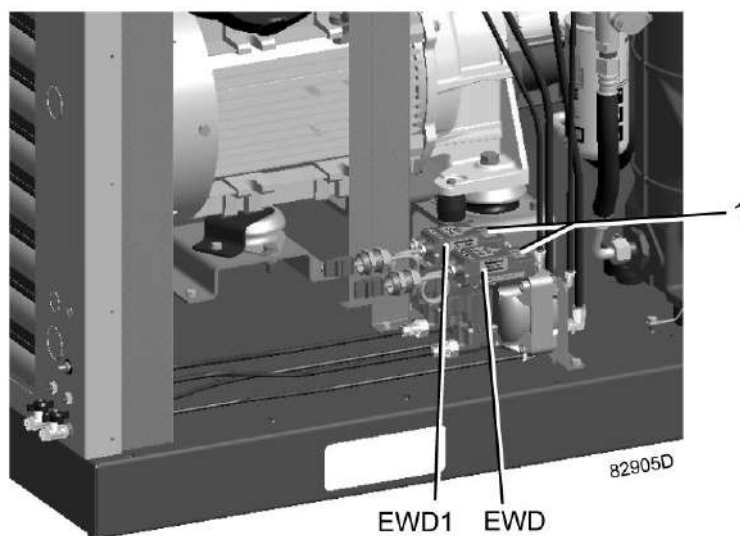
Электронные блоки дренажа конденсата, типовой пример
