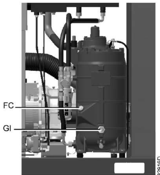
Расположение смотрового стекла уровня масла
