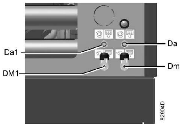
Клапаны для дренажа конденсата, типичные примеры
