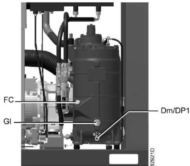
Заглушки сливного и маслналивного отверстий в сосуде маслоотделителя
