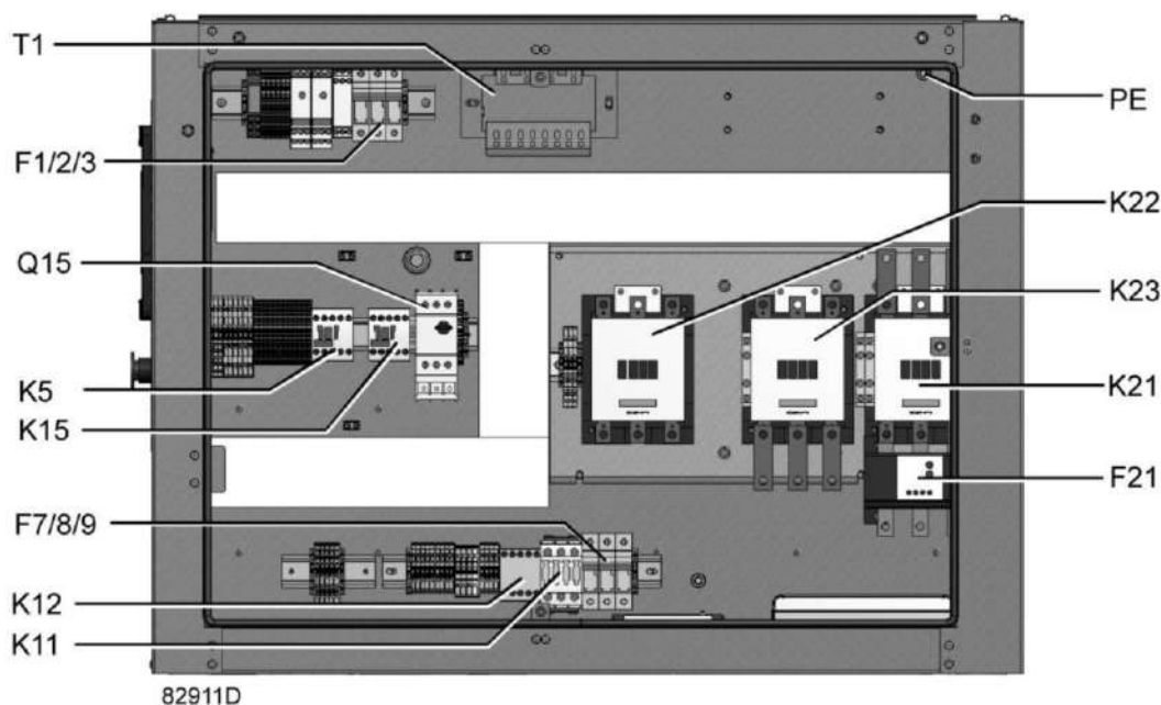
Типичный пример электрического шкафа компрессоров с GA 30+ по GA 45+
