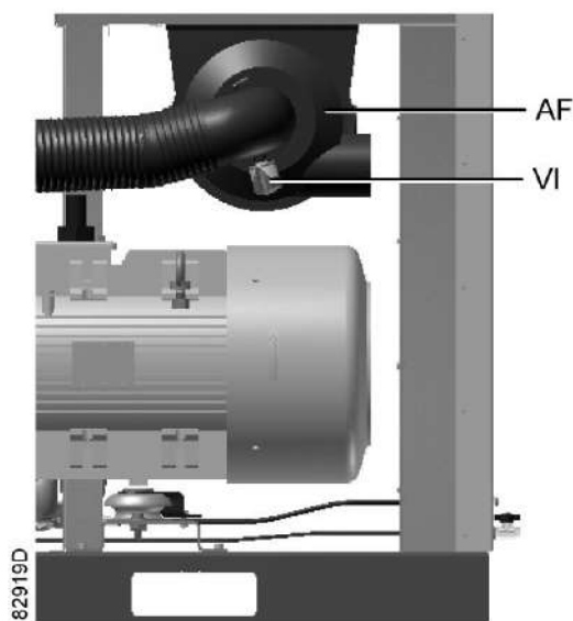
Положение воздушного фильтра и сервисного индикатора.
