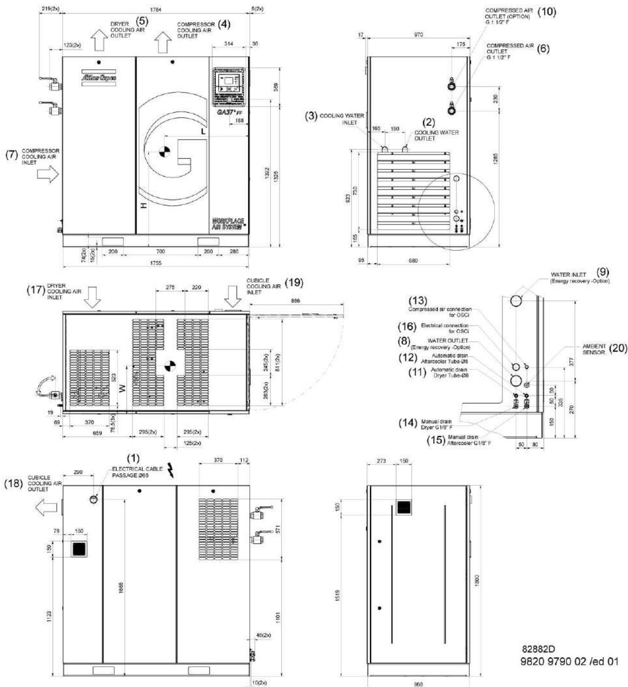
Габаритные размеры компрессоров GA 30+ – GA 45+
