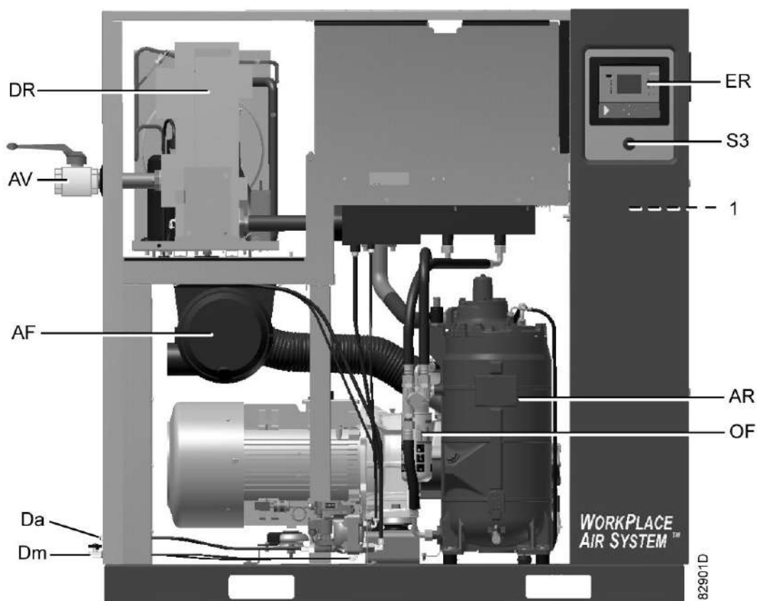
Вид спереди, компрессоры с GA 30+ по GA 45+ Full-Feature
