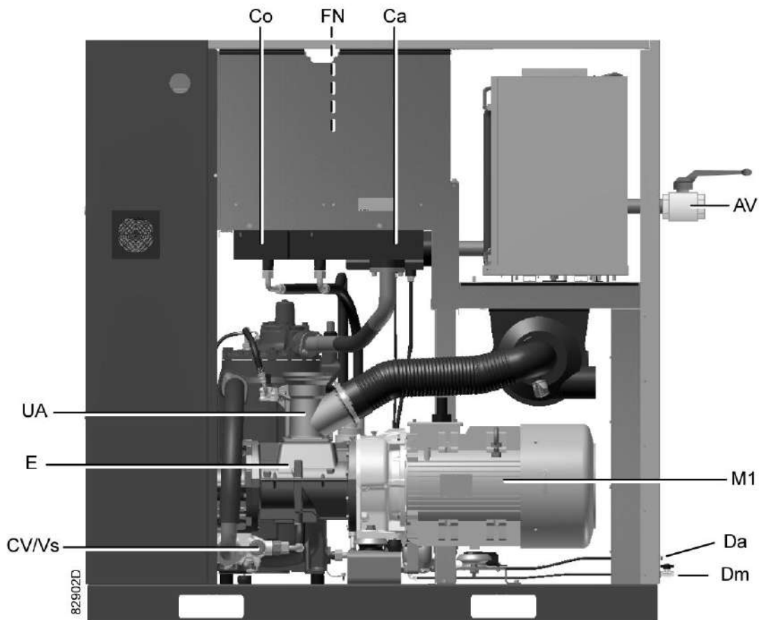
Вид сзади, компрессоры с GA 30+ по GA 45+ Full-Feature
