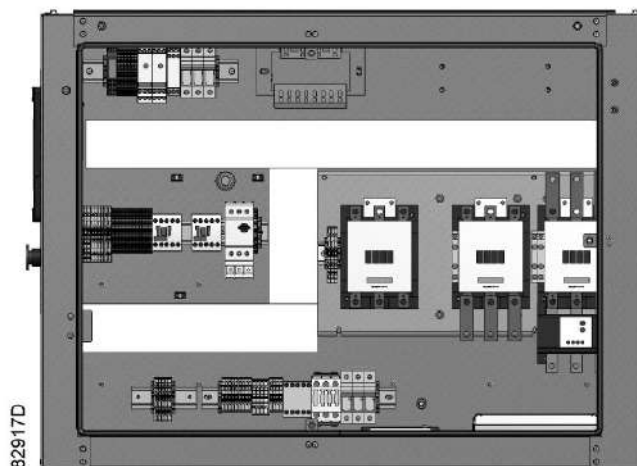
Электрический шкаф компрессоров с GA 30 + по GA 45 (типовой)
