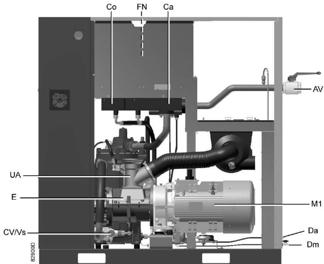
Вид сзади, компрессоры с GA 30 + по GA 45 +
