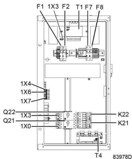
Электрический шкаф SF 8 + и SF 11 + , типовой
