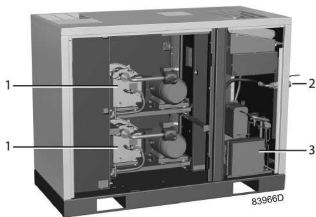
SF 8+ FF, модификация с низким корпусом, вид сзади
