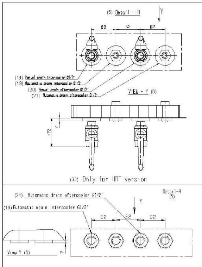
Размерный чертеж компрессоров ZR 400/500 VSD, страница 2
