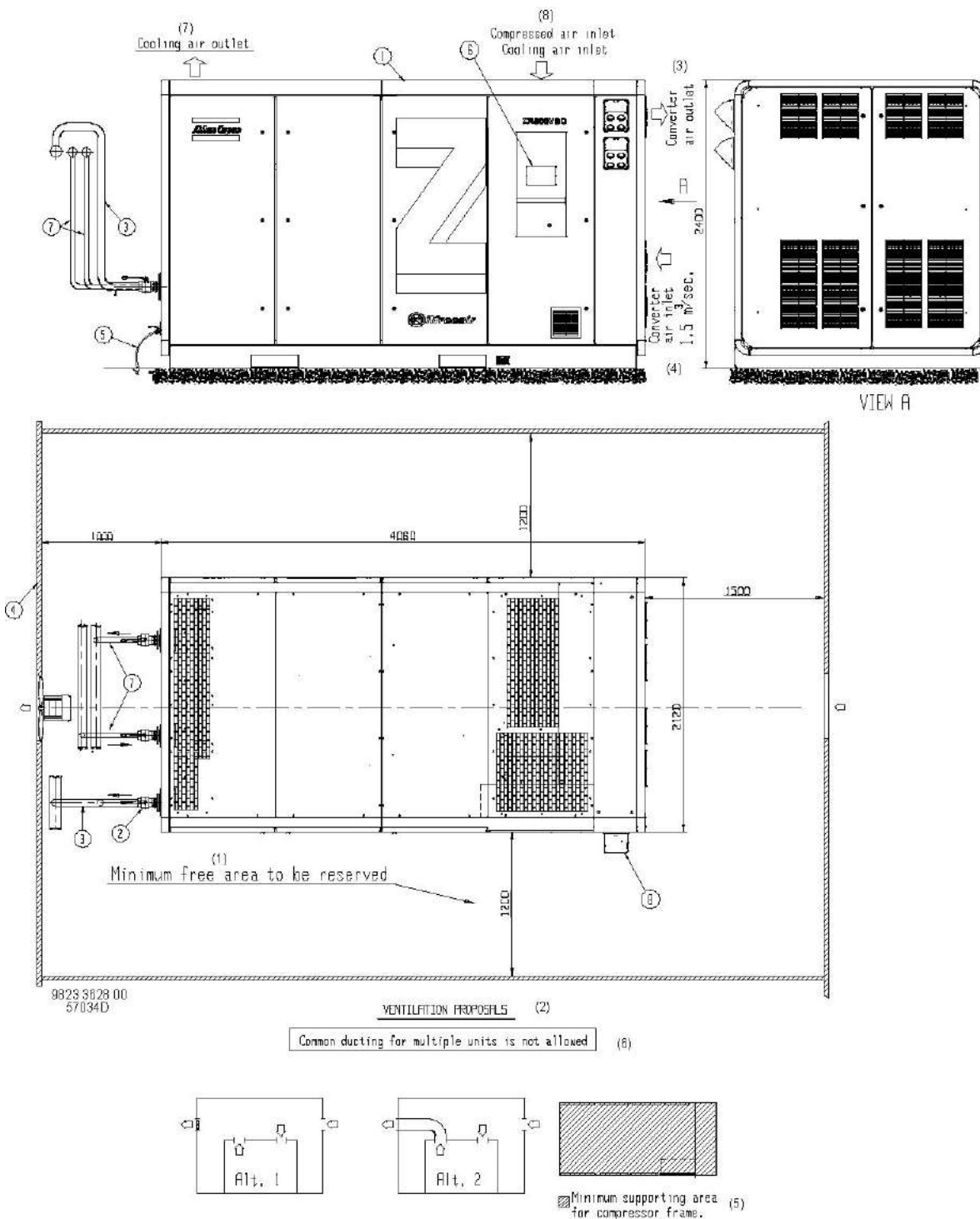
Рекомендации по установке компрессоров ZR 400/500 VSD
