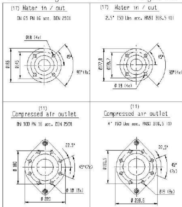
(22) DIN - flanges
