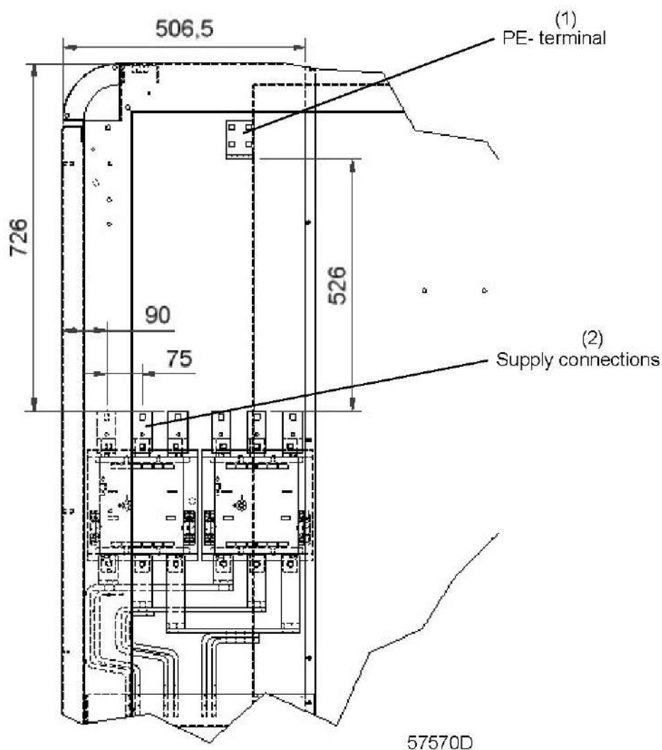
Вид шкафа управления компрессора ZR 400/500 VSD спереди
