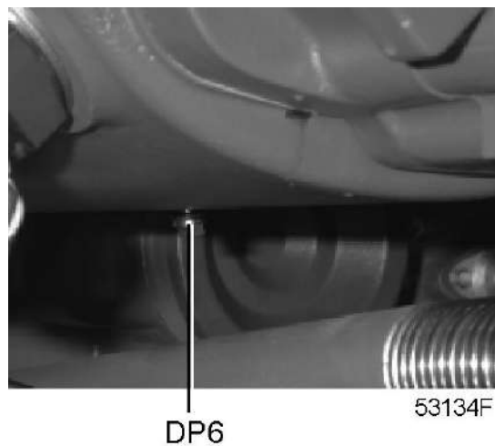
Заглушка дренажного отверстия, элемент низкого давления
