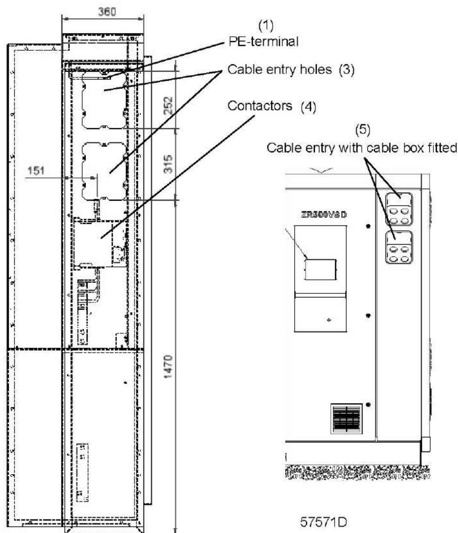
Вид шкафа управления компрессора ZR 400/500 VSD сбоку (со стороны входа кабеля)
