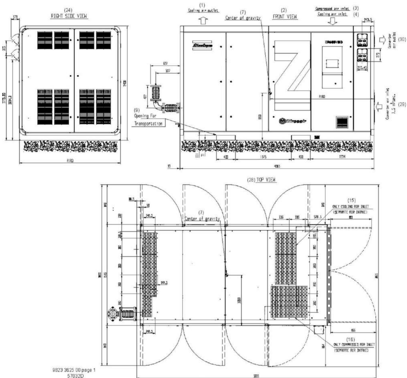
Размерный чертеж компрессоров ZR 400/500 VSD, модификация с использованием нагретого воздуха, страница 1
