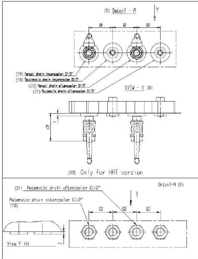
Размерный чертеж компрессоров ZR 400/500 VSD с системой рекуперации энергии, страница 2
