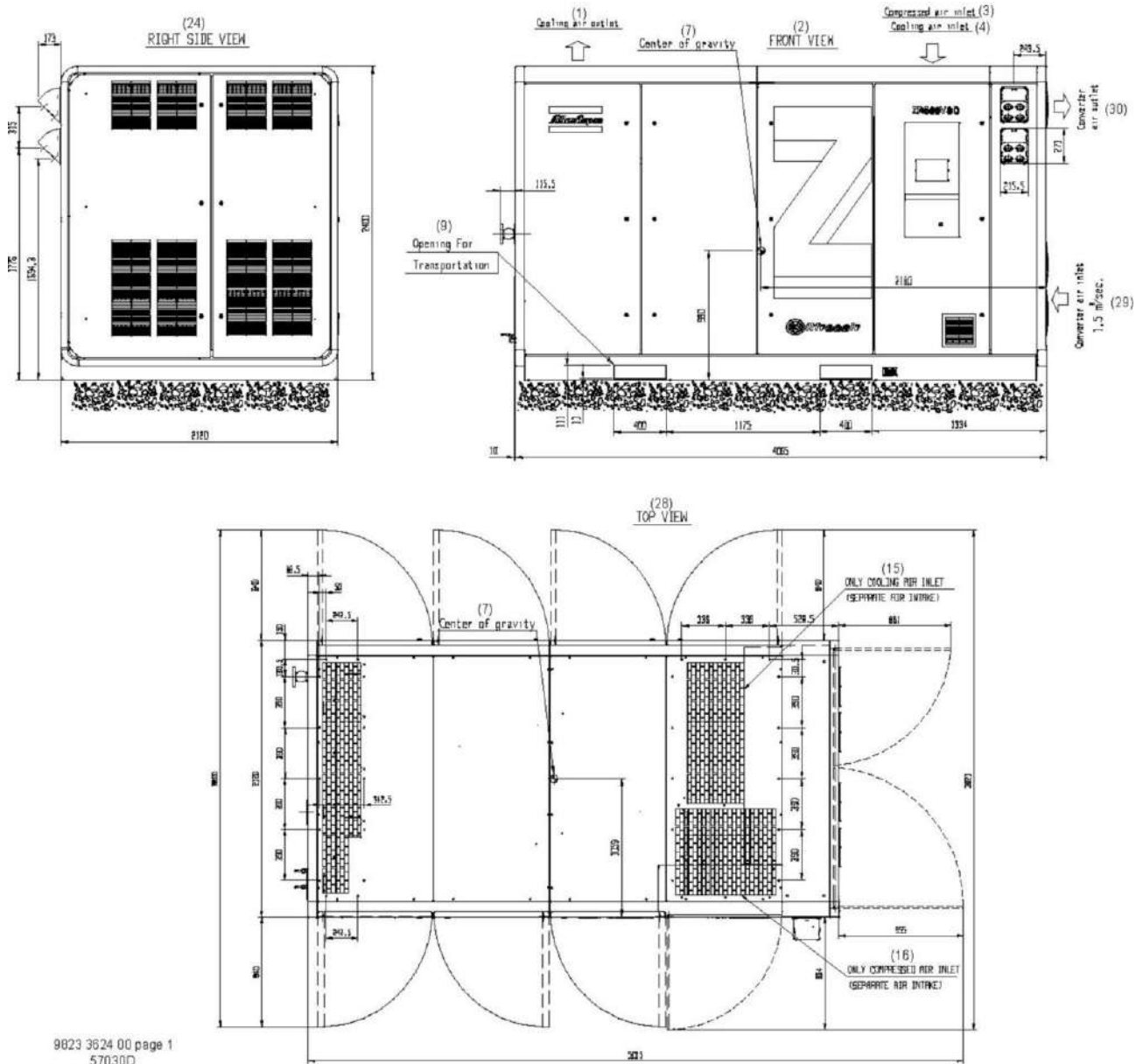
Размерный чертеж компрессоров ZR 400/500 VSD с системой рекуперации энергии, страница 1
