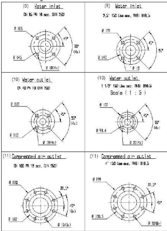
(22) DIN-Flanges
