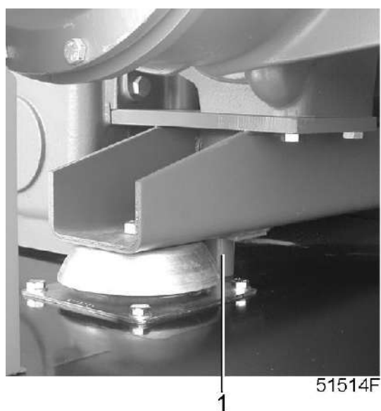
Транспортировочные крепления на стороне корпуса редуктора/охладителя компрессоров ZR 400/500 VSD
