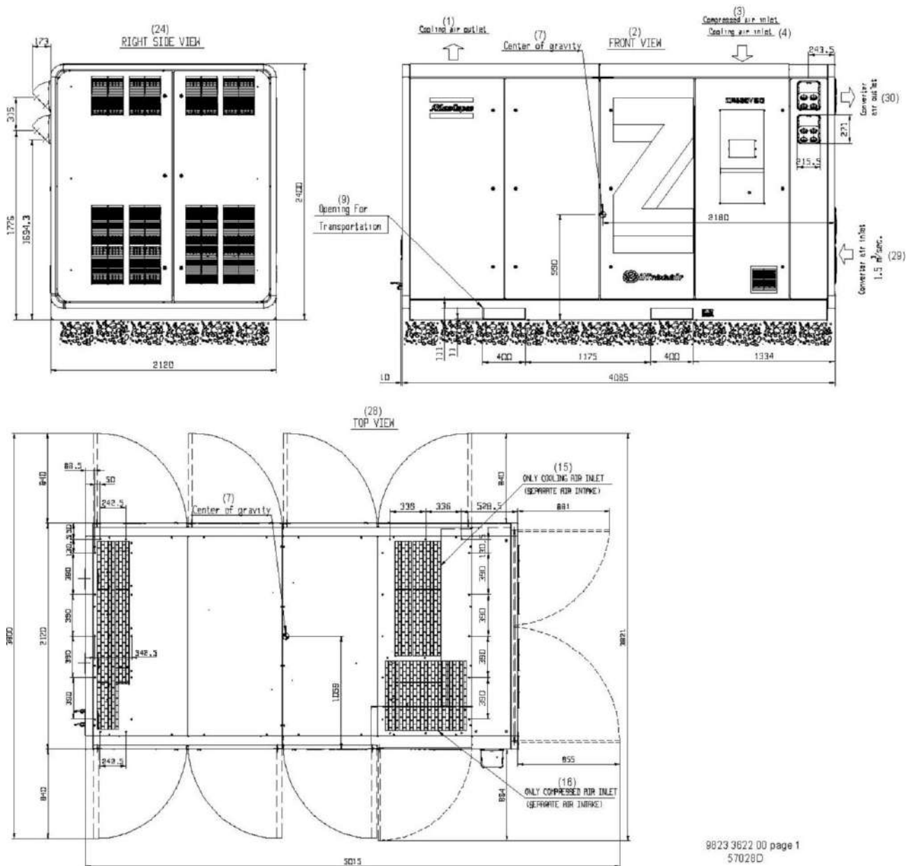
Размерный чертёж компрессоров ZR 400/500 VSD, страница 1
