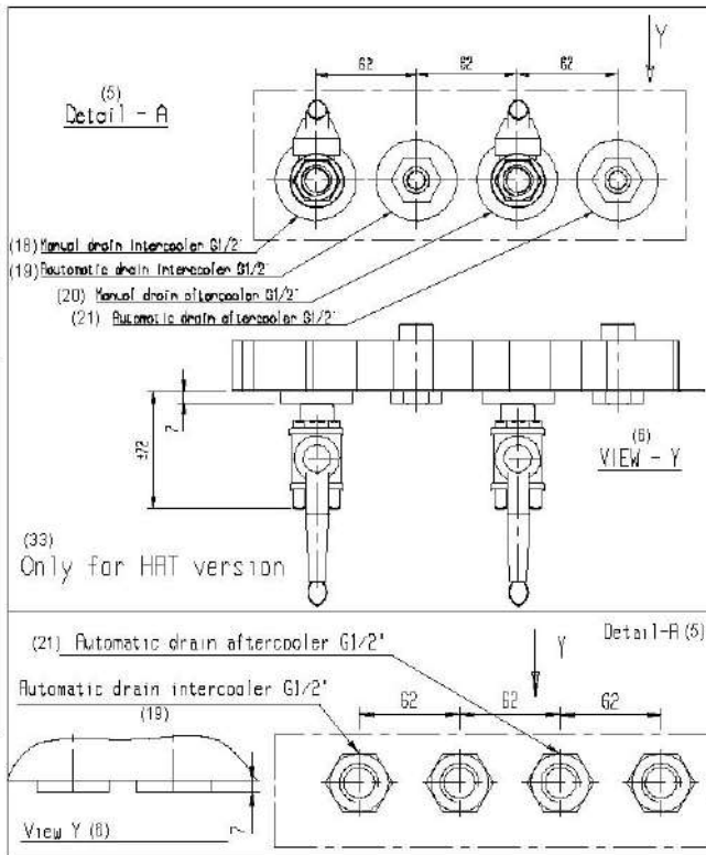
Размерный чертеж компрессоров ZR 400/500 VSD, модификация с использованием нагретого воздуха, страница 2
