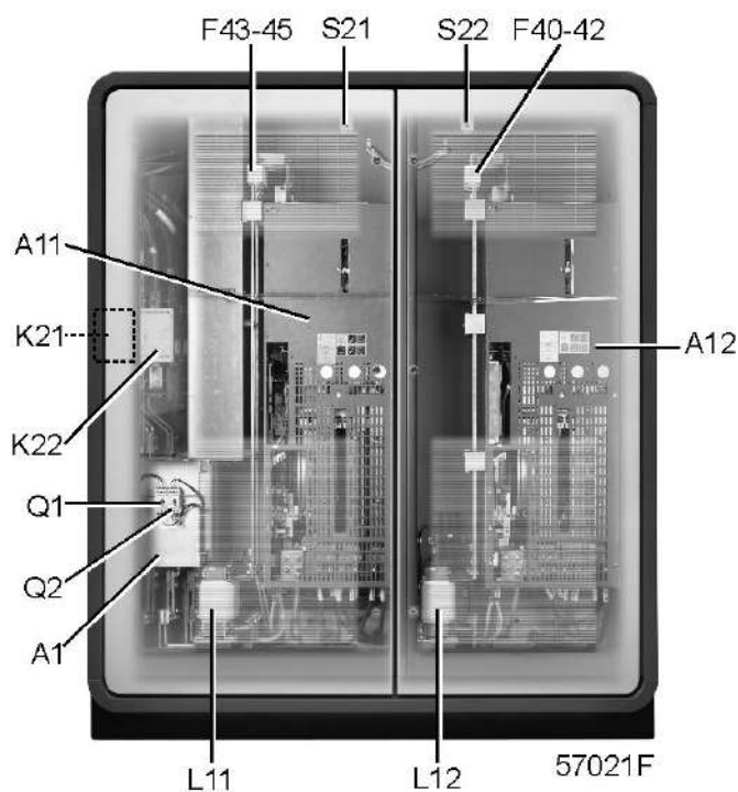
Электрический шкаф ZR 400/500 VSD
