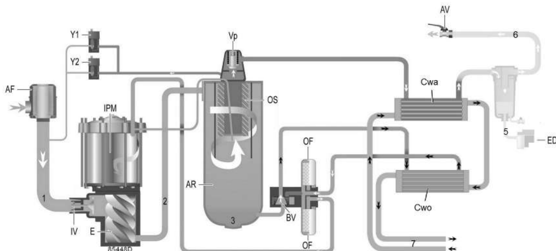
Система охлаждения, компрессоры с водяным охлаждением
