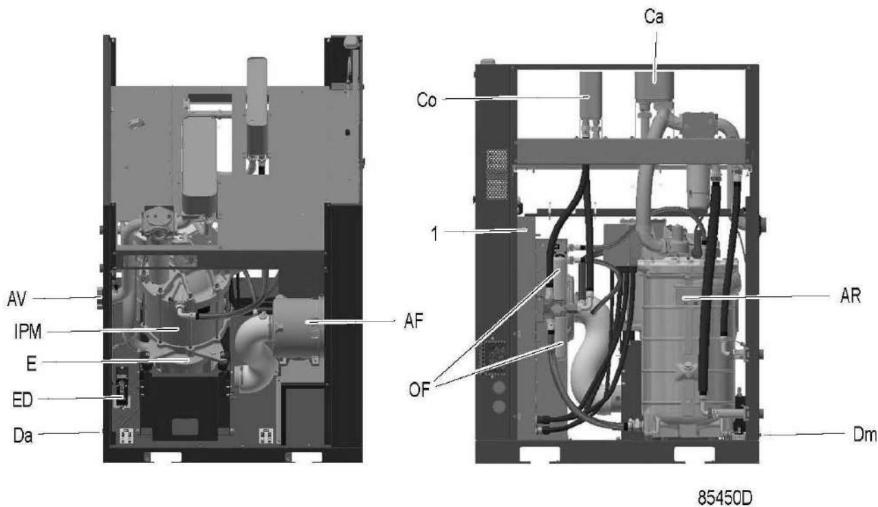
Открытый вид сбоку, GA VSD+ Pack
