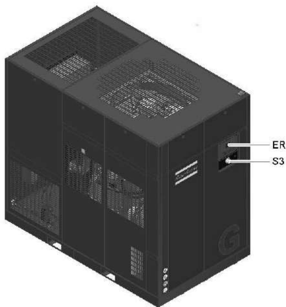
Вид спереди, GA VSD+ Full-Feature
