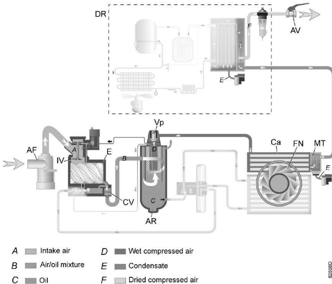
Схема потока, компрессоры GA Workplace Full-Feature
