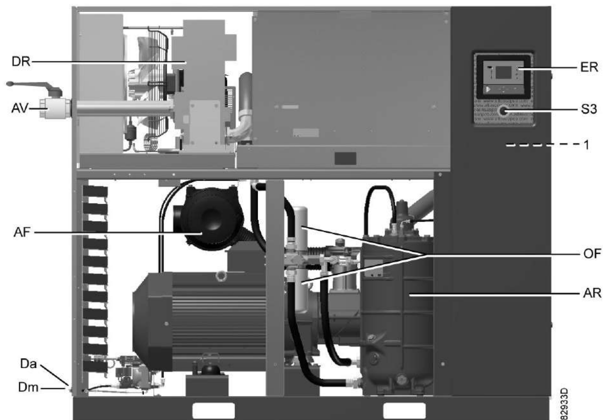
Вид спереди, компрессоры с GA 55+ по GA 90 Full-Feature
