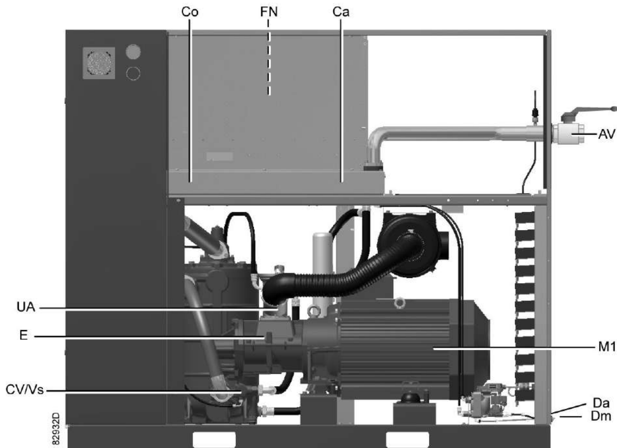
Вид сзади, компрессоры с GA 55+ по GA 90
