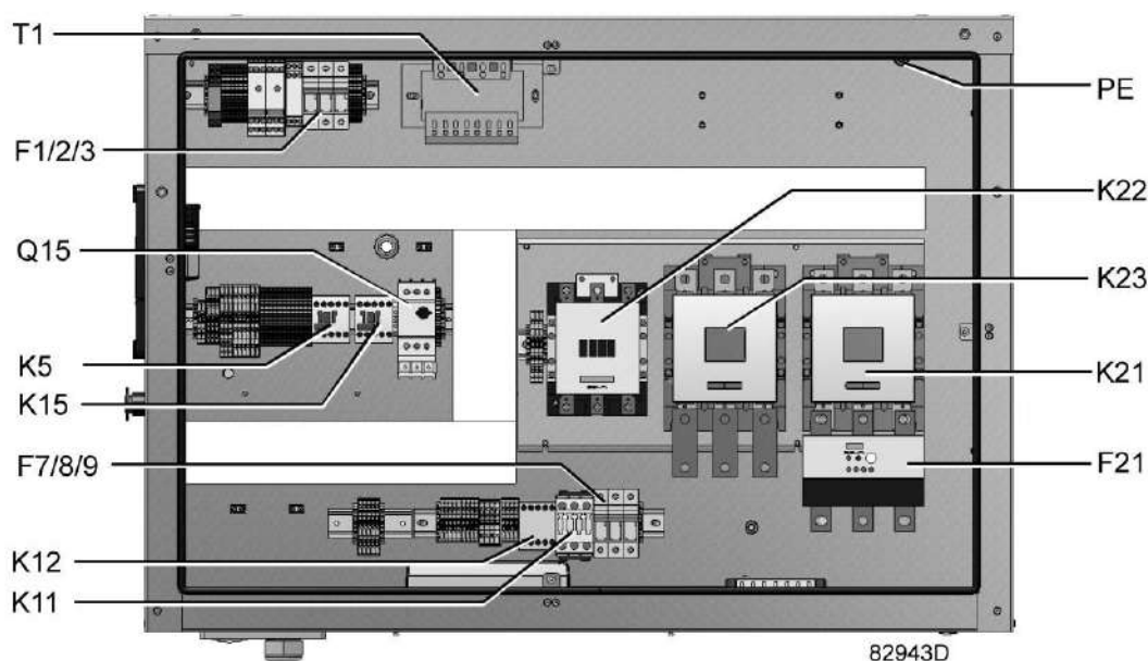
Типичный пример электрического шкафа компрессоров с GA 55+ по GA 90
