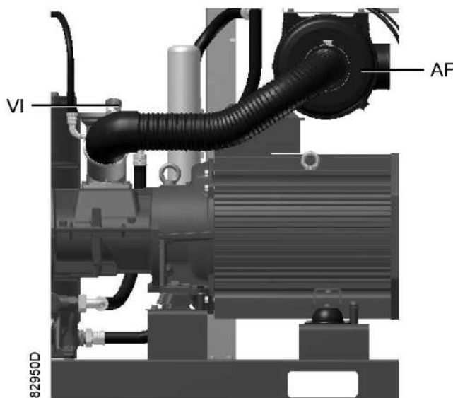
Положение воздушного фильтра и сервисного индикатора.
