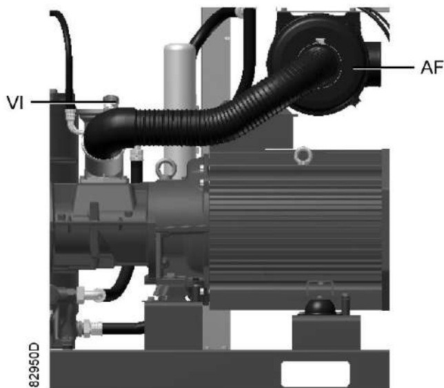
Расположение сервисного индикатора
