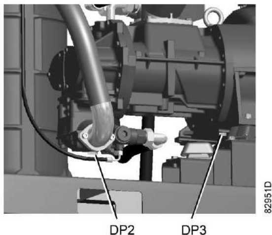
Заглушки сливных отверстий, обратный клапан и корпус редуктора
