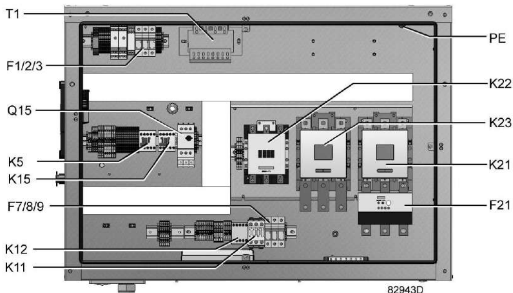
Пример электрического шкафа компрессоров с GA 55+ по GA 90
