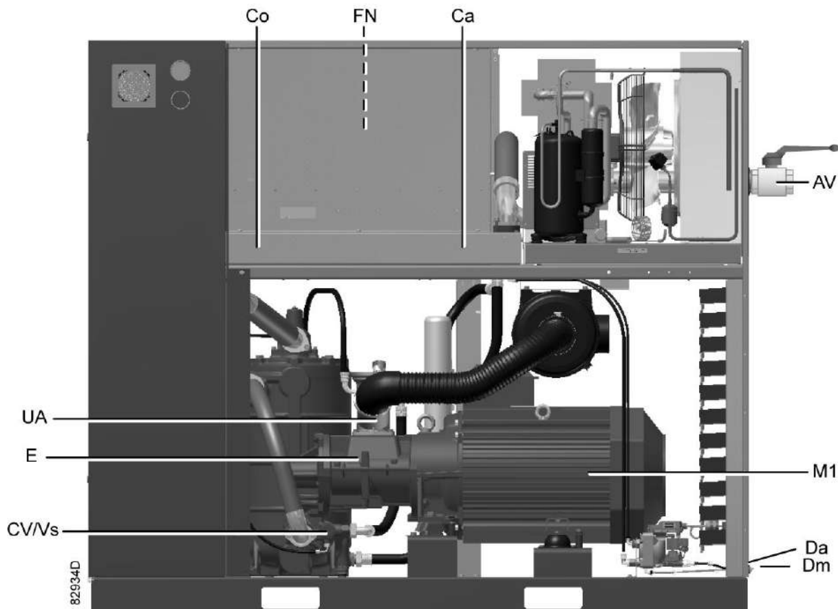
Вид сзади, компрессоры с GA 55 + по GA 90 Full-Feature
