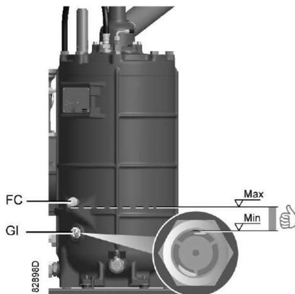
Расположение смотрового стекла уровня масла
