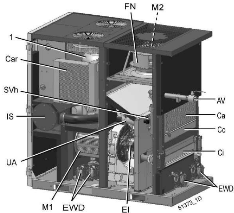
Вид сзади, Full-Feature (осушитель IMD)
