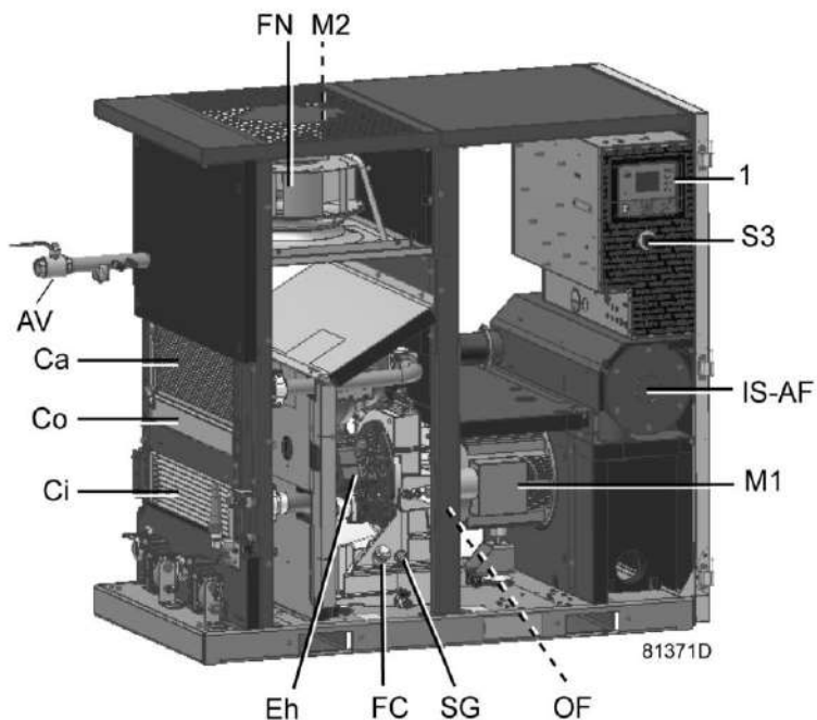
Вид спереди, Pack
