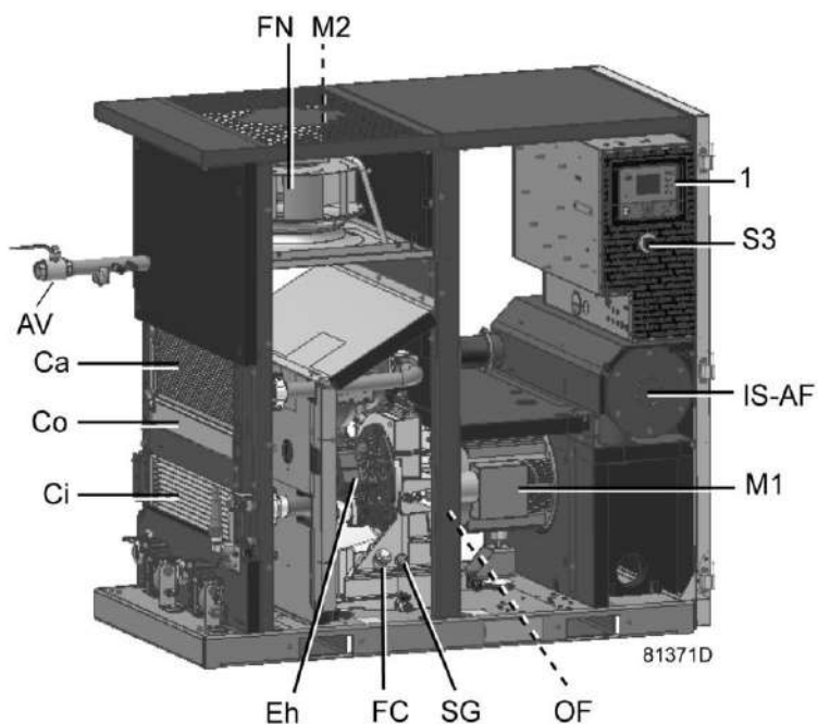
Расположение воздушного фильтра
