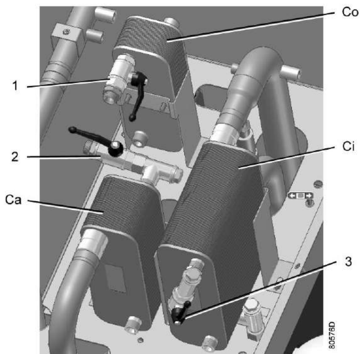
Охладители и водяные клапаны (ZR)
