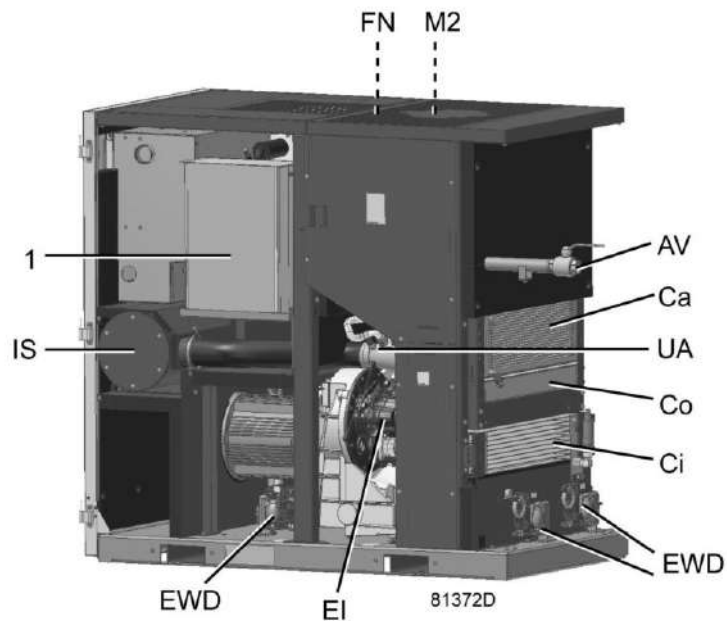
Вид сзади, Full-feature (осушитель ID)
