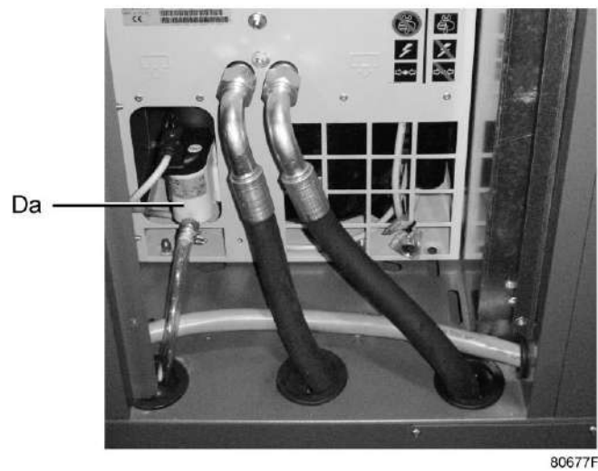
Дренаж конденсата
