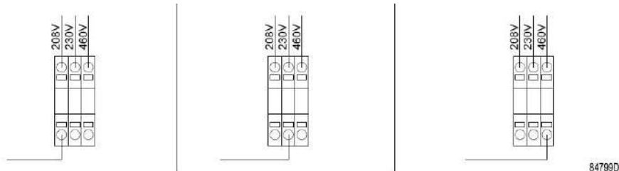
Клемма осушителя X5
