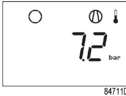
Основной экран с индикацией останова и выходной температуры компрессорного элемента
